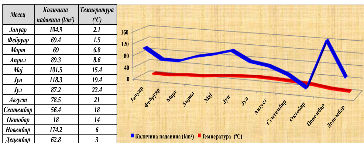
Слика 5.4. Дијаграм количине падавина и температуре ваздуха за 2023. годину
