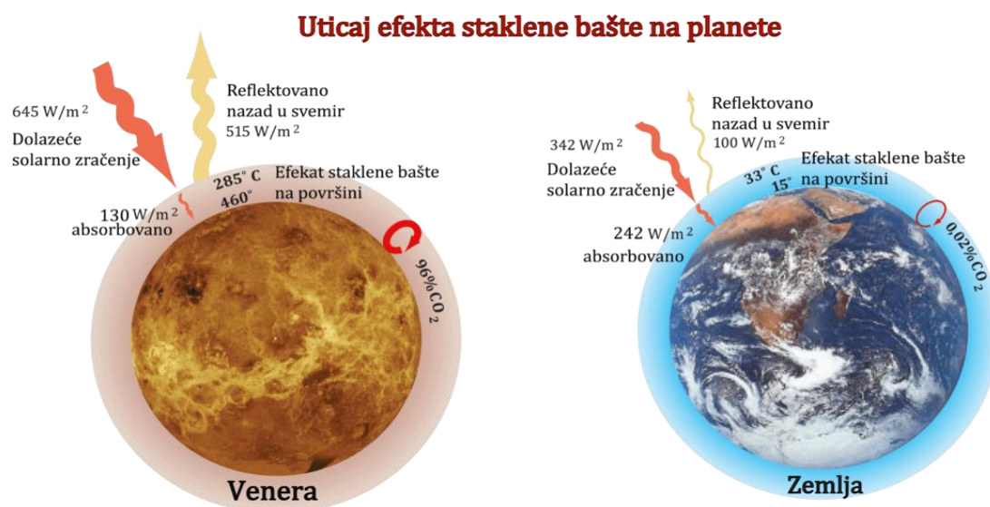
Слика 5.5. Ефекат стаклене баште
