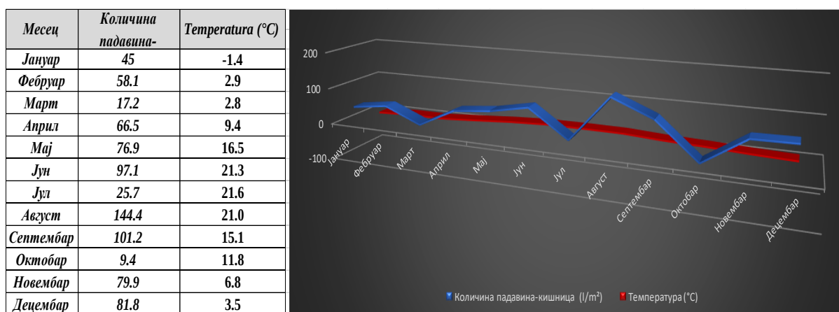
Слика 5.3. Дијаграм количине падавина и температуре ваздуха за 2022. годину
